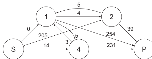
Figure 12 - Exemple de graphe résiduel
