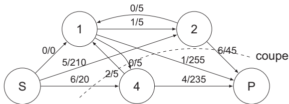
Figure 13 - Coupe dans un graphe
