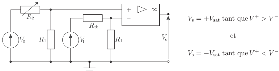
FIGURE 2 – Montage à amplificateur linéaire
